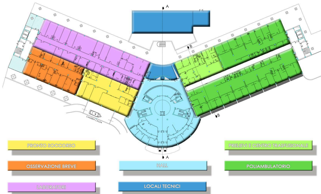
PIANTA PIANO TERRENO
