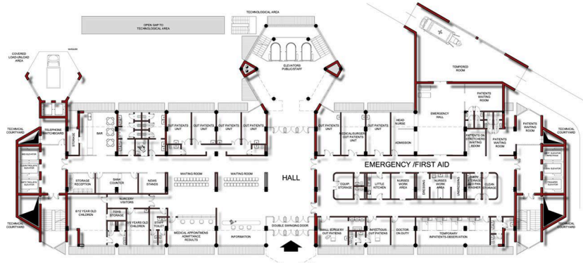
PLAN REZ DE CHAUSSEE
