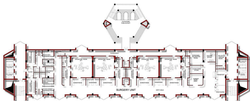
PLAN DES SALLES D'OPÉRATION
