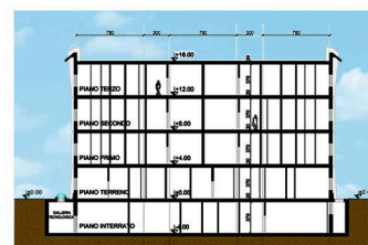
COUPE B-B
