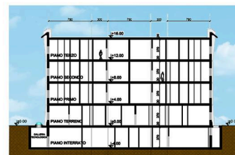
SEZIONE B-B
