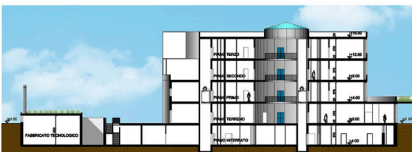
SEZIONE A-A
