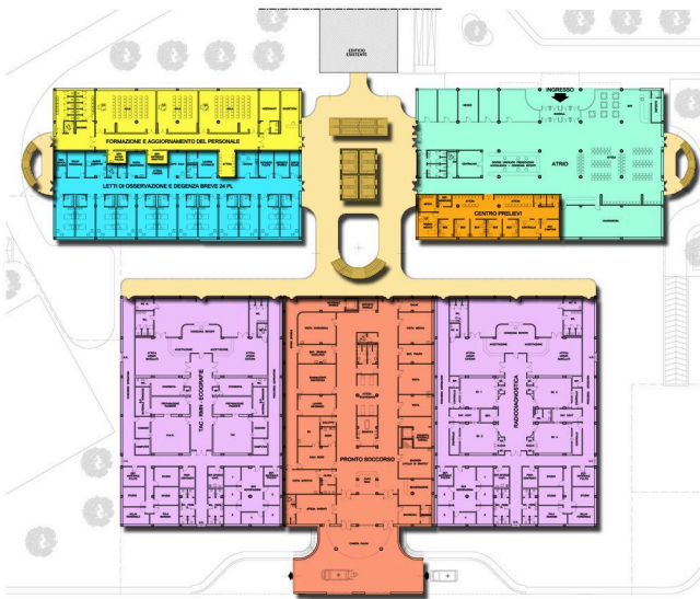
PLAN REZ DE CHAUSSEE
