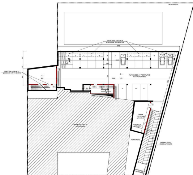
PIANTA PIANO INTERRATO
