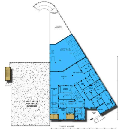
FABBRICATO TECNOLOGICO - PIANTA PIANO TERRENO
