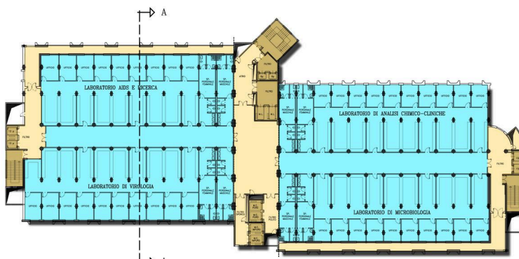
PIANTA PIANO SESTO
