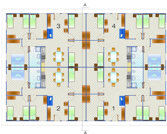
MODULO DA QUATTRO UNITÀ ABITATIVE Appartamenti da 85 mq
