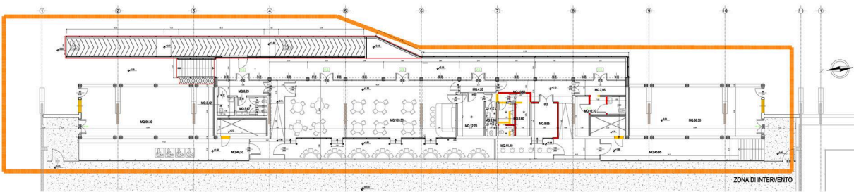
ÉCOLE D'ÉQUITATION - PLAN REZ DE CHAUSSÉE
