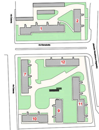
PLANIMETRIA GENERALE
