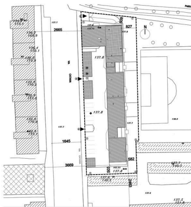
PLANIMETRIA GENERALE
