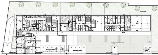
PIANTA PIANO TERRENO
