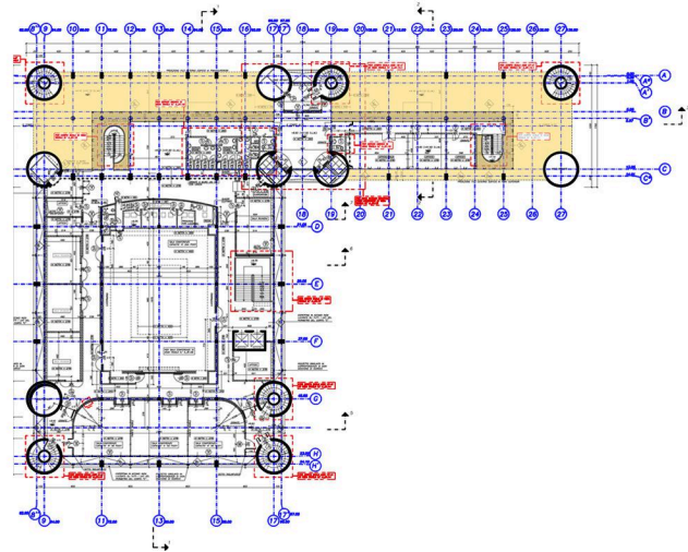
PLAN DU MEZZANINE
