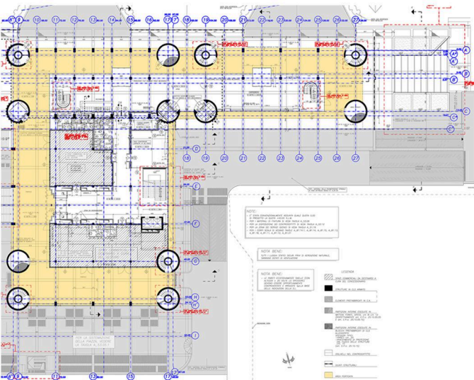
PLAN REZ DE CHAUSÉE
