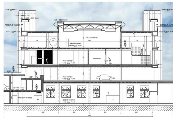
SEZIONE TRASVERSALE
