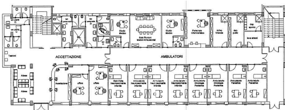
BÂTIMENT B - PLAN REZ DE CHAUSSÉE
