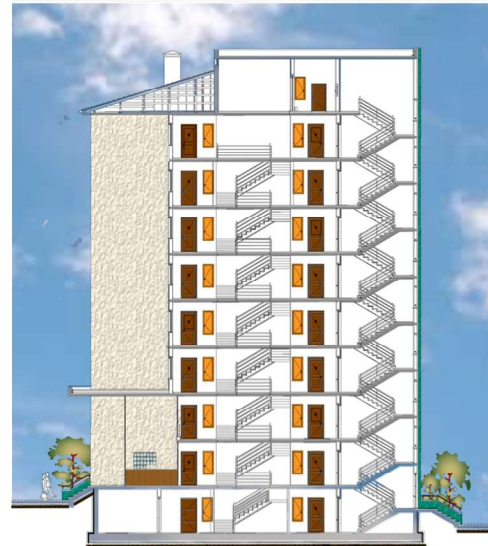
COUPE B-B
