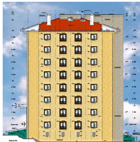
FAÇADE LATÉRALE
