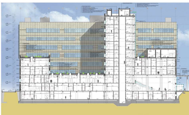
LONGITUDINAL SECTION 1-1
