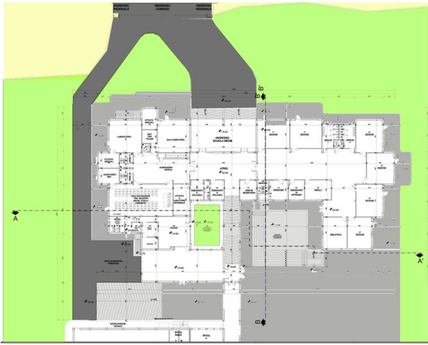
PLAN REZ DE CHAUSSÉE
